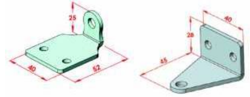
Bağlantı Parçaları
